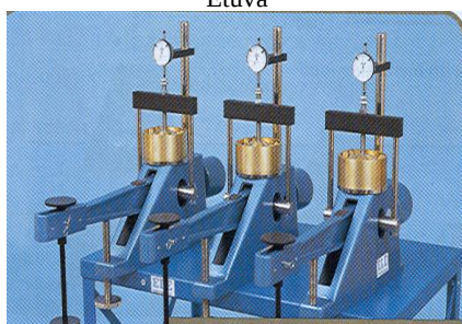
Edometru cu trei posturi (compresiune - consolidare)
